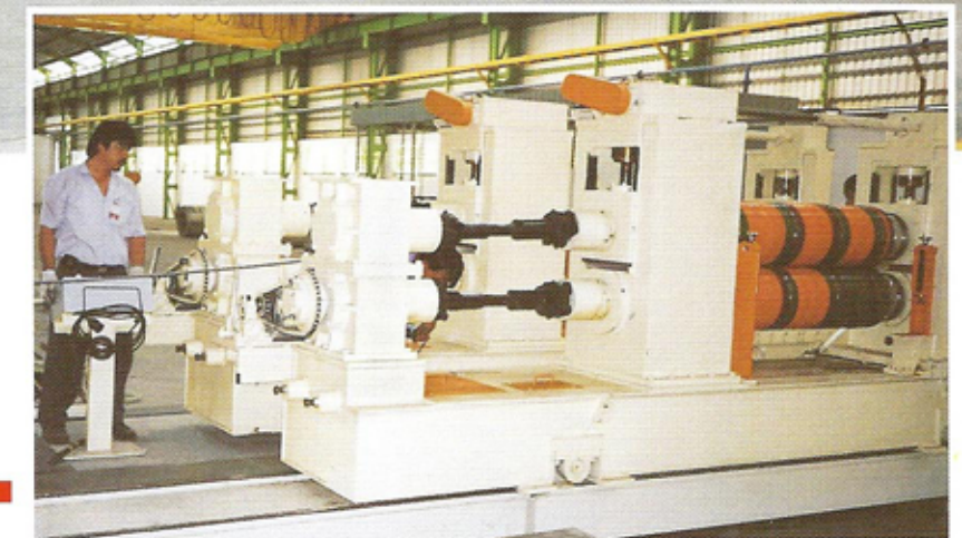
台車交換式雙刀座 ■ TWO EXCHANGEABLE SLITTER CARTS
