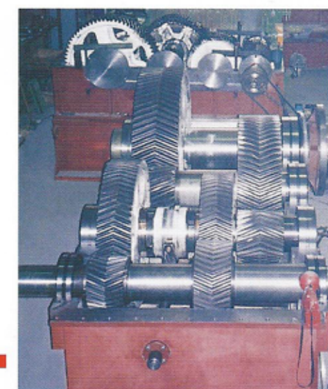
■ 強力齒輪箱，高扭力、低噪音 POWERFUL GEARBOX, HIGH TORQUE, LOW NOISE
