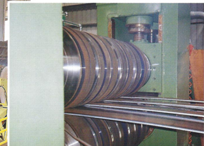
■ 高精度分條主機 HIGH PRECISION SLITTER
