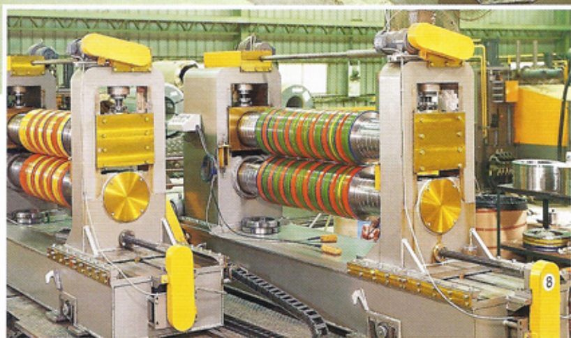
■ 台車交換式雙刀座 TWO EXCHANGABLE SLITTER CARTS
